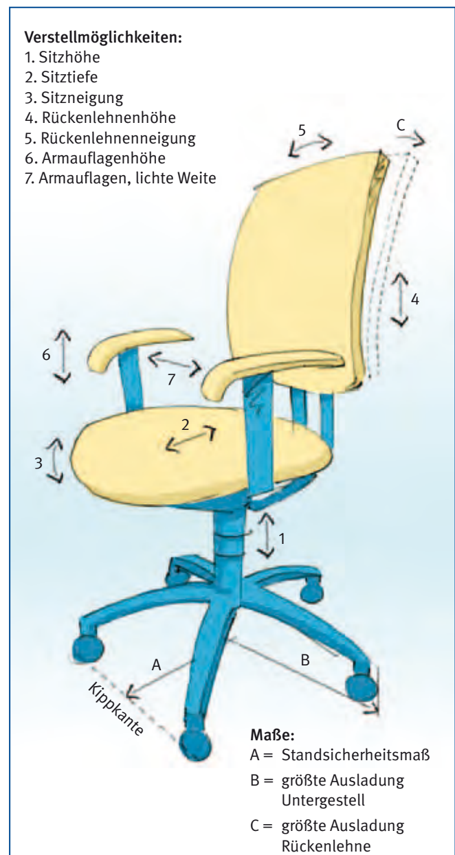
Abbildung 35: Büroarbeitsstuhl
